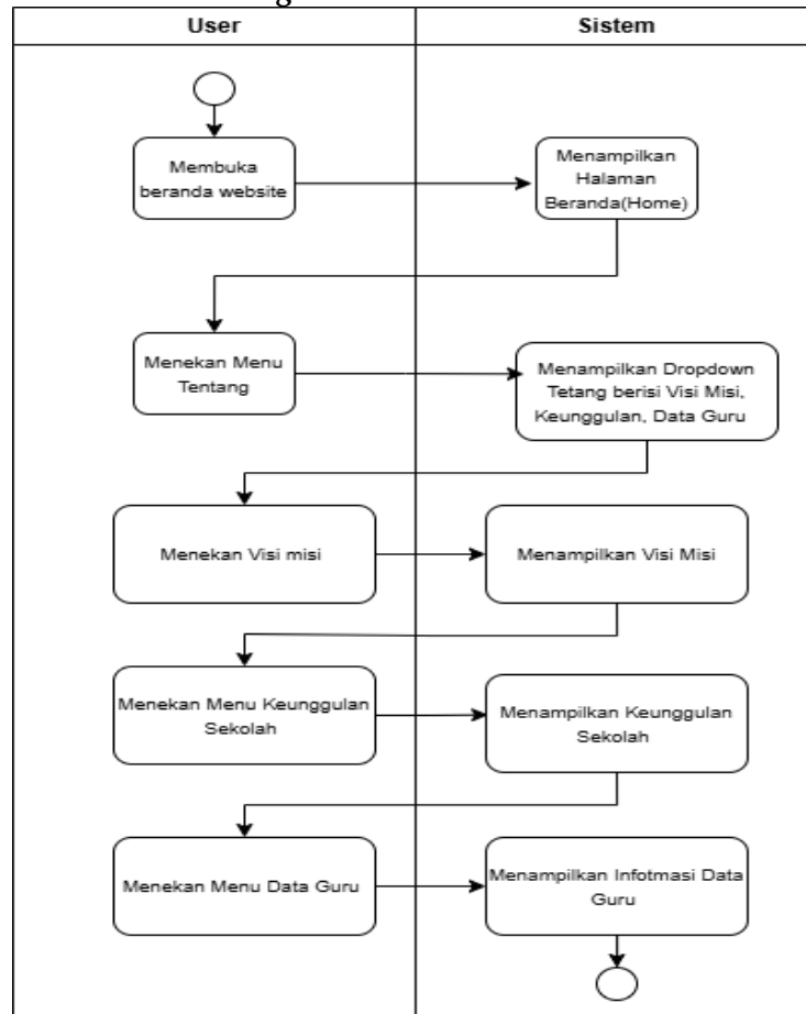
Gambar 2. Activity Diagram User Melihat Tentang Kami
